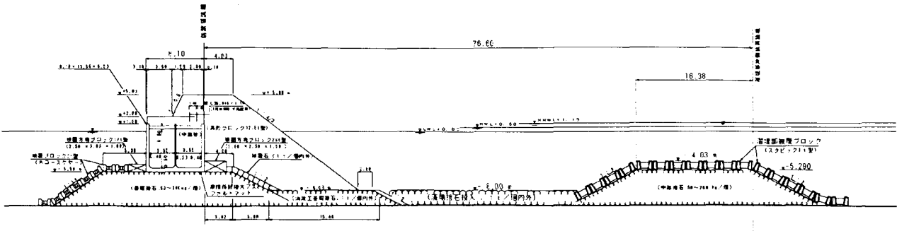
図-1 藻場造成型防波堤の標準断面
