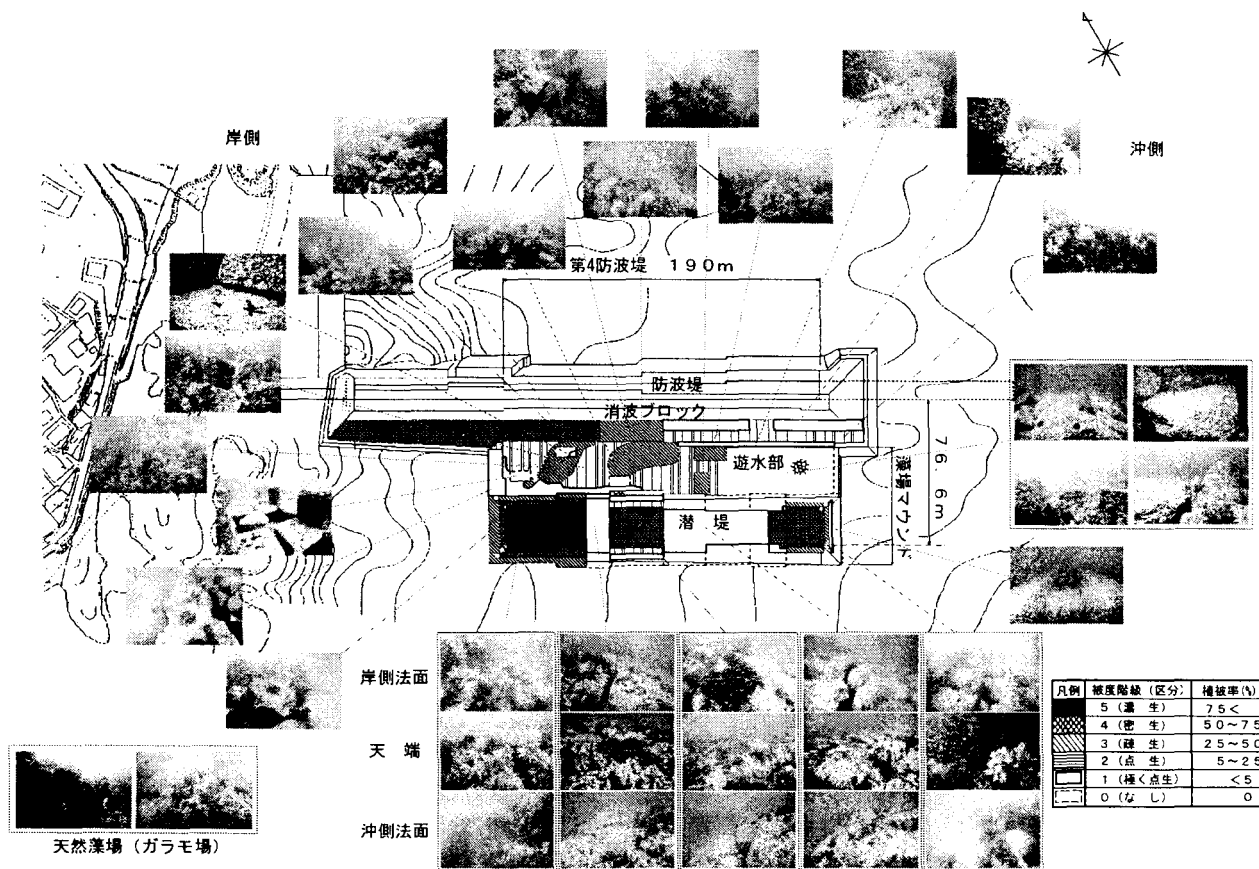
図-7 富来漁港 藻場造成型防波堤の藻場分布図 (平成15年3月)
