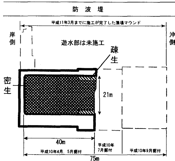
図-3 平成11年3月の藻場分布
